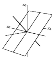
Subspaces Nul A and Row A
