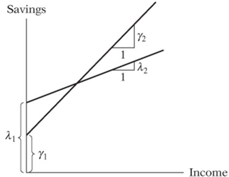
(d) Dissimilar regressions
