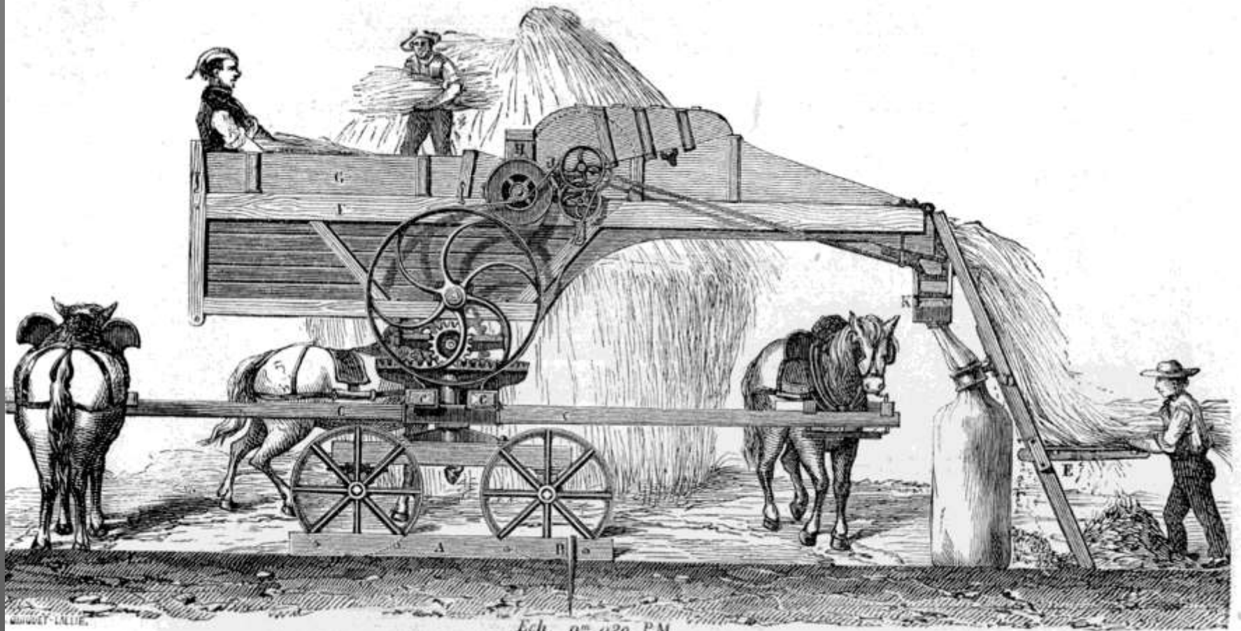
Ech. 0m 020 P.M. Fig. 349. — Batteuse Damey à manège direct placé sous la batteuse.
